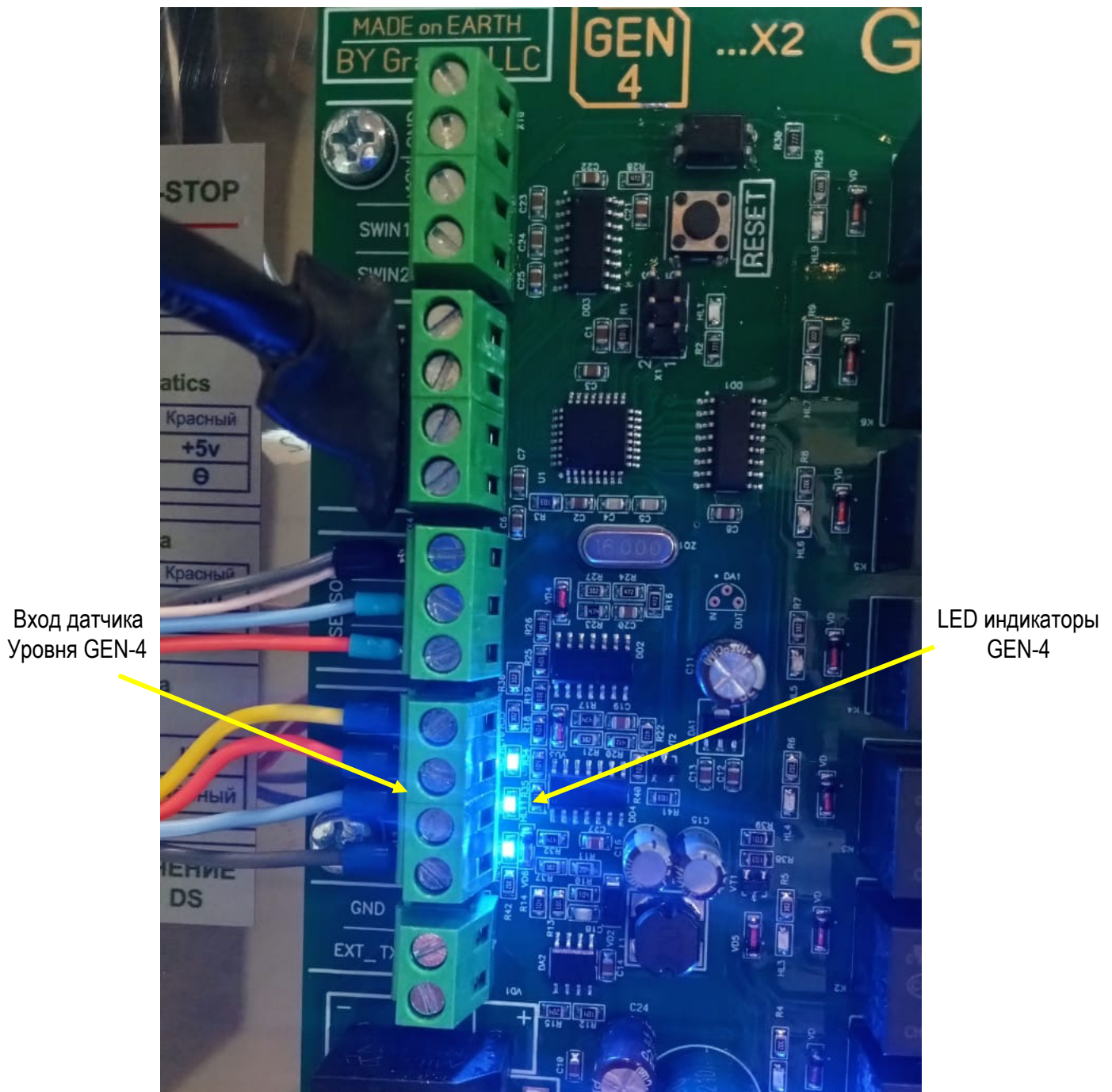
Фото платы и LED индикаторов
