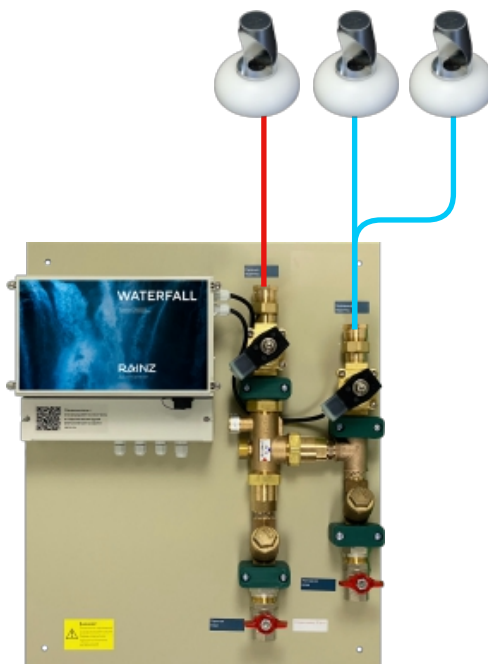
Схема подключения: одна форсунка теплого водопада + две форсунки холодного водопада
