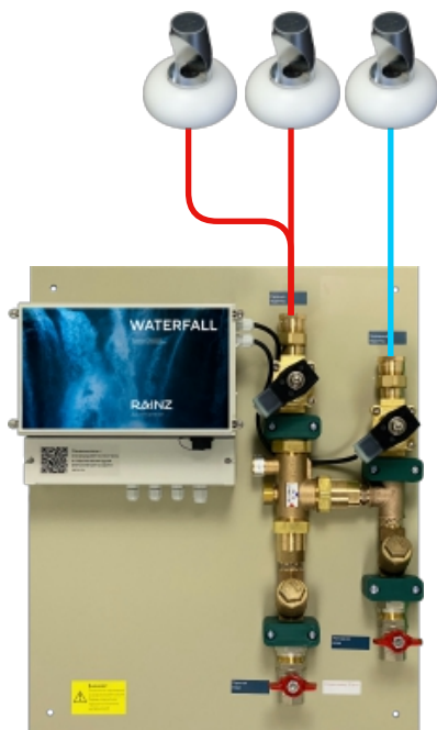
Схема подключения: две форсунки теплого водопада + одна форсунка холодного водопада
